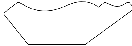
KL 312 .750 x 2.250 1.875 1.313
