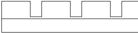
KL 340 .500 x .625
