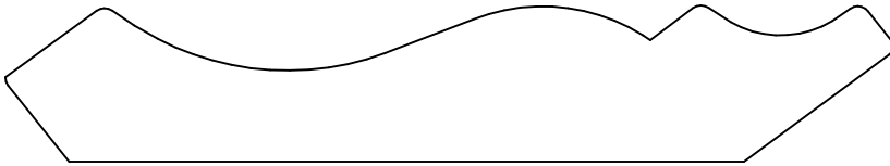
KL 314 .750 x 4.250 3.500 2.438
