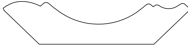
KL 307 .750 x 3.250 2.313 2.313
