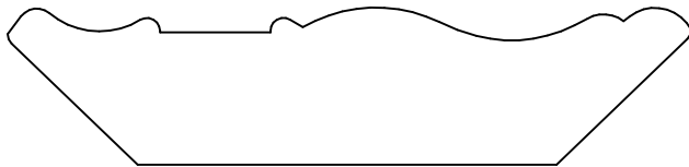
KL 1363 .750 x 3.250 2.313 2.313
