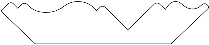
KL 341 .750 x 3.625 2.625 2.563
