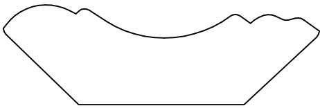
KL 306 .750 x 2.375 1.688
