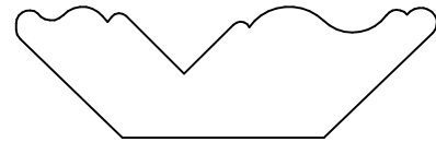
KL 377 .625 x 2.000 1.438 1.500
