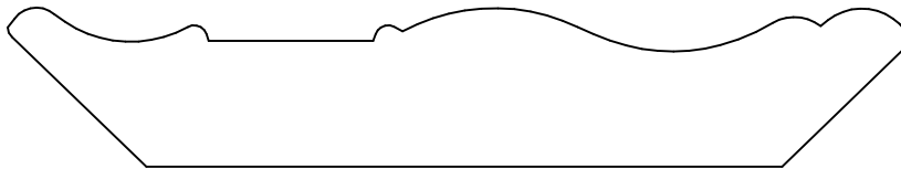
KL 1364 .750 x 4.250 3.063 3.000
